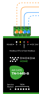
Шлюз ONOKOM TN-1-MB-B
