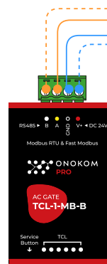
Шлюз ONOKOM TCL-1-MB-B
