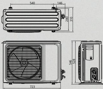
Модель: AL-H12/4R1B(U)
