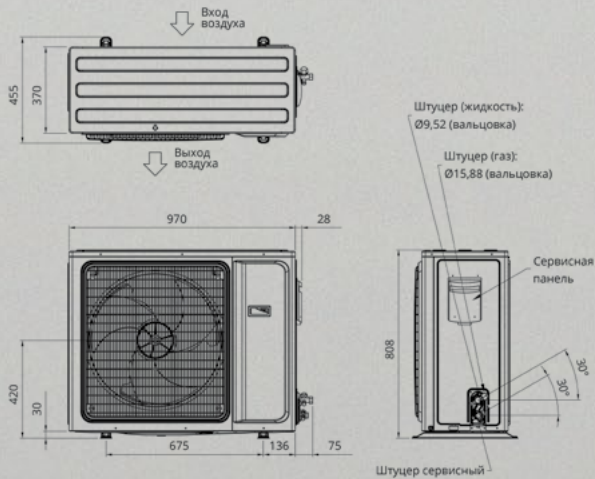
Модель: AL-H36/5R1B(U)
