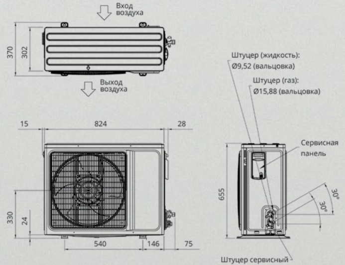
Модель: AL-H24/4R1B(U)
