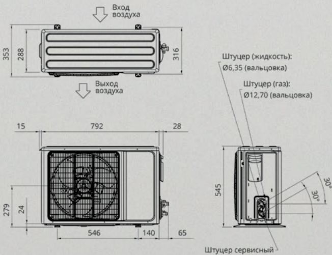
Модель: AL-H36/5R1B(U)
