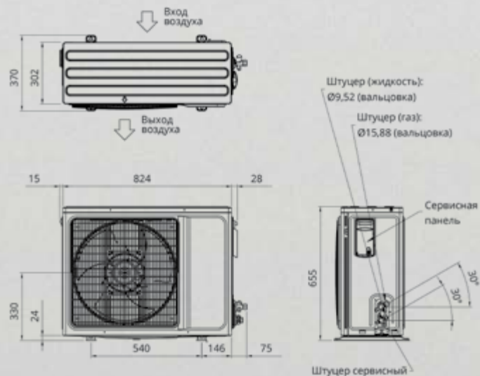
Модель: AL-H24/4R1B(U)-v1
