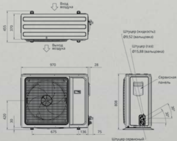
Модель: AL-H36/5R1B(U)-v1
