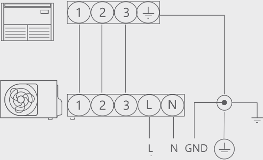
Электрическая схема (опциональная)
