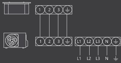
Электрическая схема (трехфазная)
