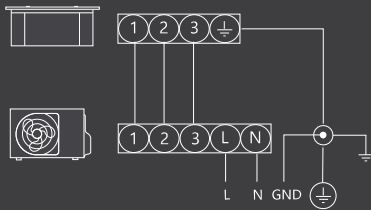
Электрическая схема (однофазная)
