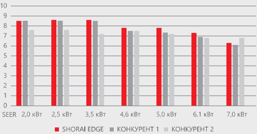
Сезонная энергоэффективность в режиме обогрева SEER
