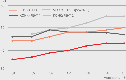
Уровень звукового давления наружных блоков, дБ(А)
