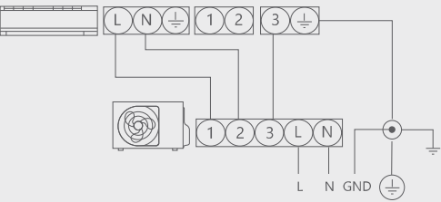
Электрическая схема (опциональная)
