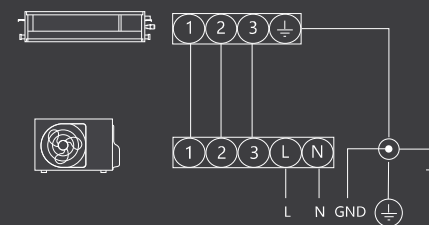
Электрическая схема
