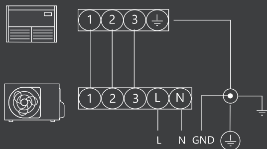
Электрическая схема (однофазная)
