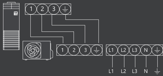
Электрическая схема (трехфазная)
