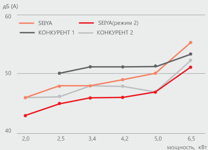
Уровень шума наружных блоков
