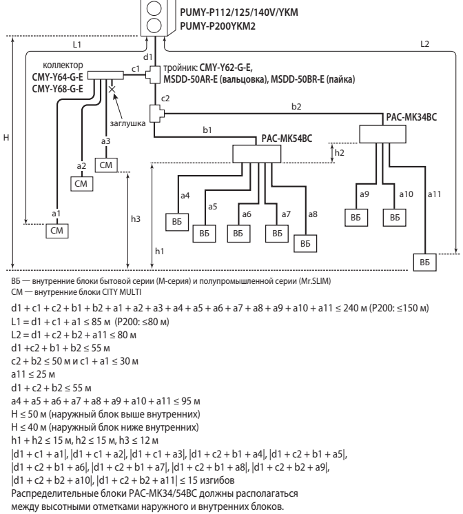
2 блока-распределителя
