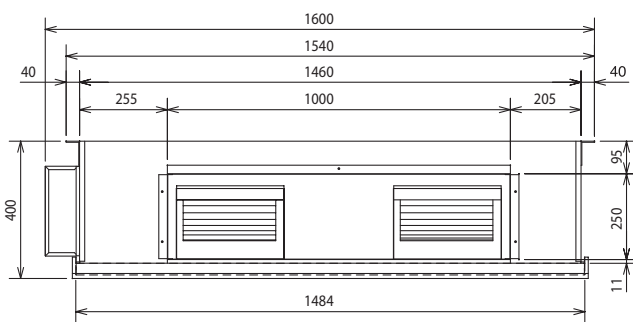
Вид спереди
