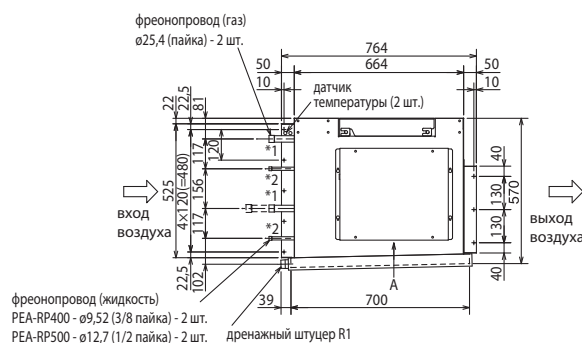
Вид слева PEA-RP400/500GAQ
