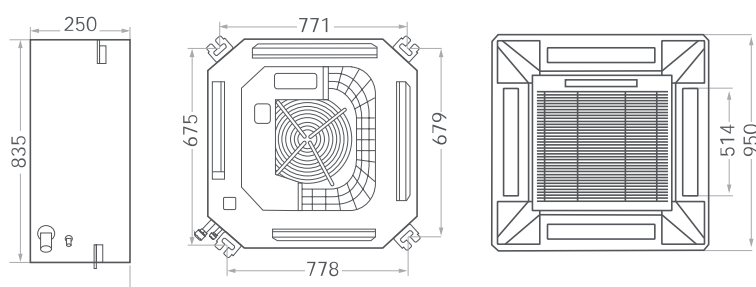
SAC48C3-A, SAC60C3-A
