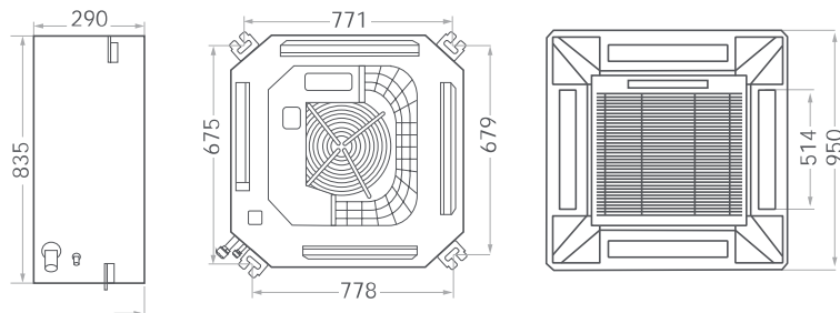
SAC48C3-A, SAC60C3-A
