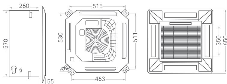
SAC24C3-A, SAC36C3-A
