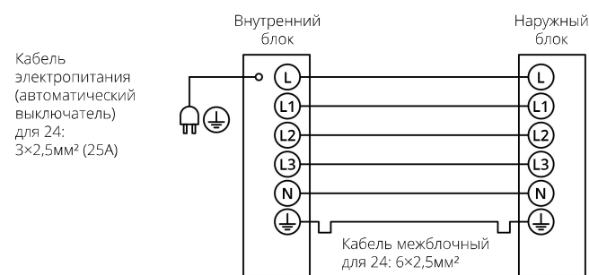
Схема подключения Elegant line On-Off (24)
