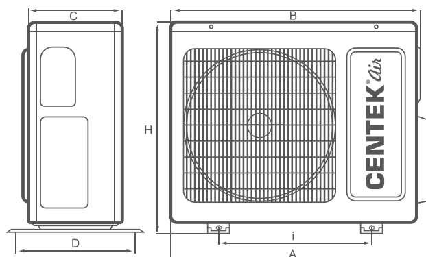
МОДЕЛЬ А, мм В, мм С, мм Д, мм Н, мм І, мм СТ-65А07+ 733 663 254 310 421 430 СТ-65А09 733 665 280 310 420 430 СТ-65А12 780 660 240 294 500 500 СТ-65А18 865 795 290 354 525 545 СТ-65А24 870 825 310 360 655 540 СТ-65А30 800 800 300 360 690 540
