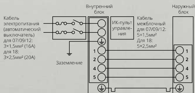
Схема подключения FJ series On-Off (24)
