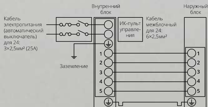
Схема подключения FJ series On-Off (24)
