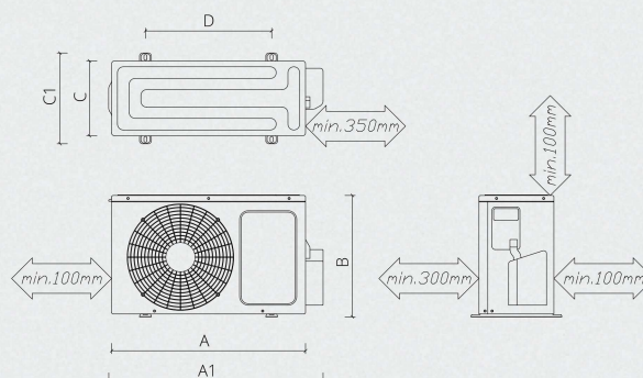
Smart inverter (LK700) наружные блоки
