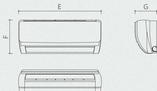
Smart inverter (LK700) внутренние блоки
